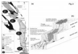
Fig. 2 : (a) : Carte géologique simplifiée, dessinée d'après les données de terrain et l'imagerie satellitaire, du massif de Closepet. Noter que le massif recoupe tout les niveaux de la croûte. 4 zones ont été distinguées (commentaire dans le texte). (b) : Bloc-diagramme indiquant les liens entre déformation et mise en place du granite à différents niveaux structuraux.
